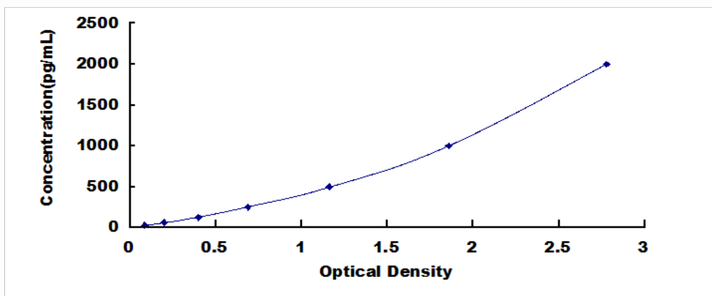
小鼠 \beta -位淀粉样前体蛋白裂解酶 1 ( \beta ACE1) 检测试剂盒标准曲线
