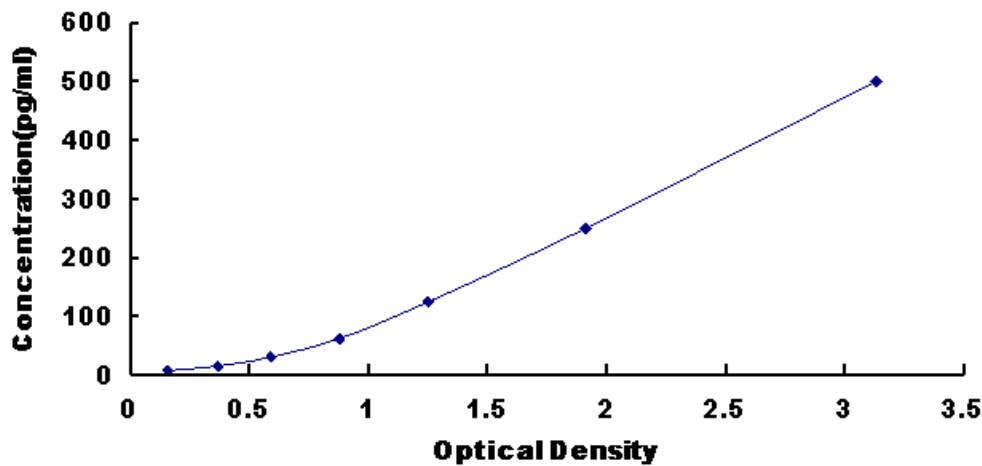
图 1: 大鼠 Dyn 试剂盒标准曲线
