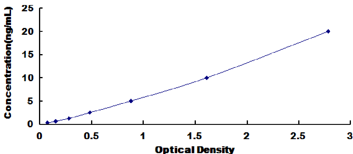
人双糖链蛋白聚糖(BGN)检测试剂盒标准曲线
