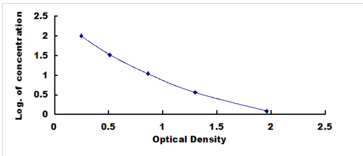
胆红素(Bb)检测试剂盒标准曲线
