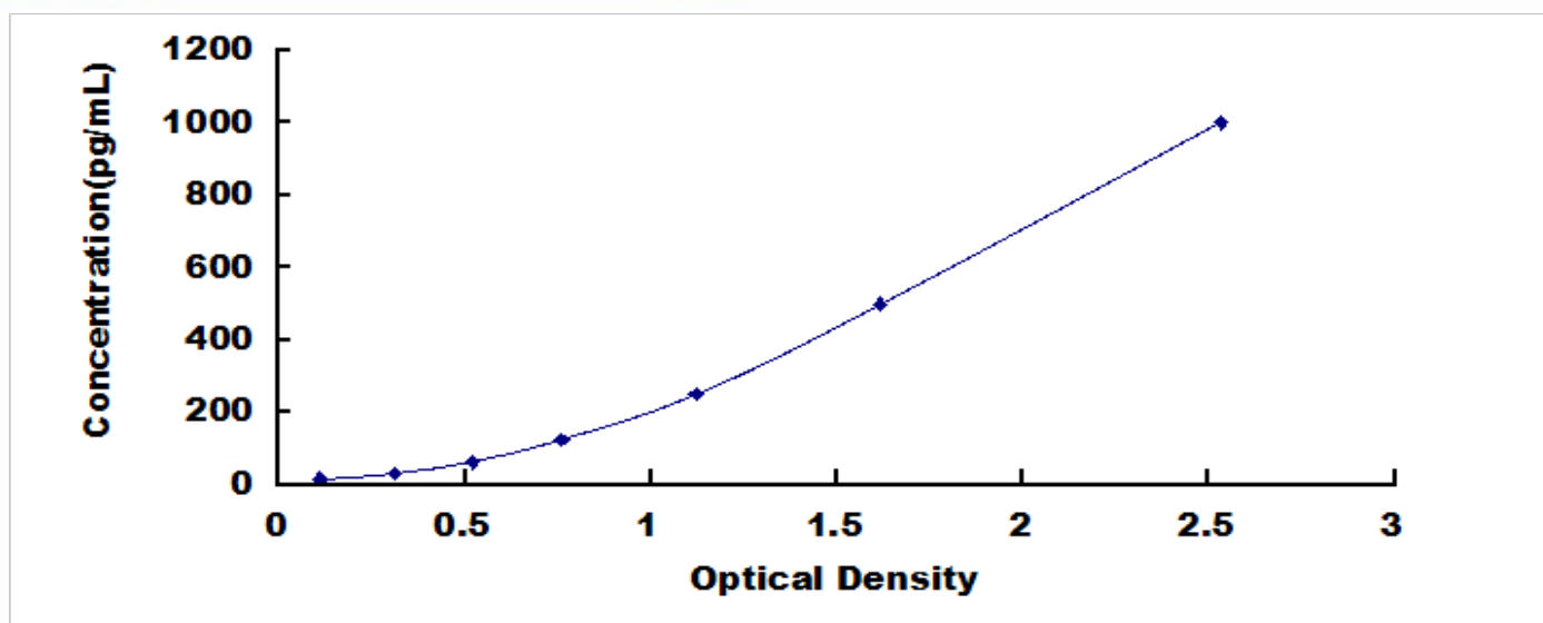
大鼠骨成型蛋白 2 (BMP2) 检测试剂盒标准曲线
