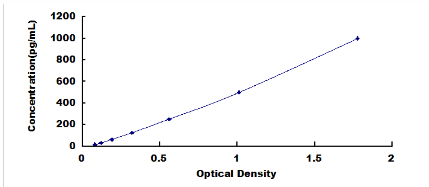
人骨形成蛋白 8B (BMP8B) 检测试剂盒标准曲线
