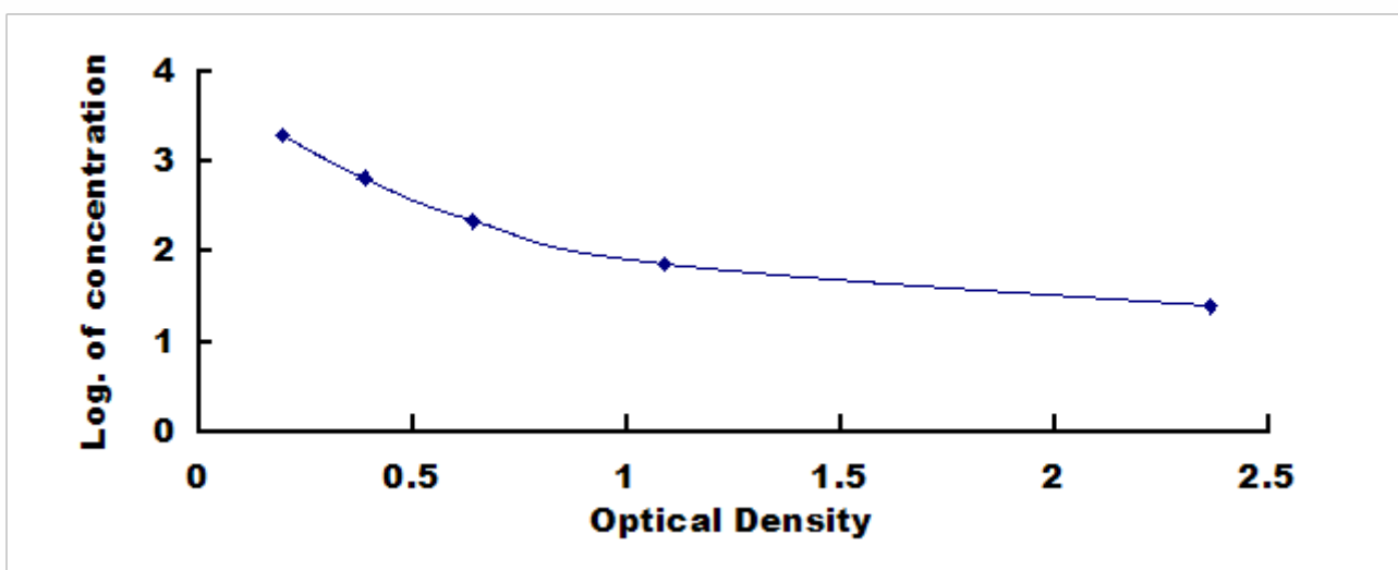
兔缓激肽(BK)检测试剂盒标准曲线
