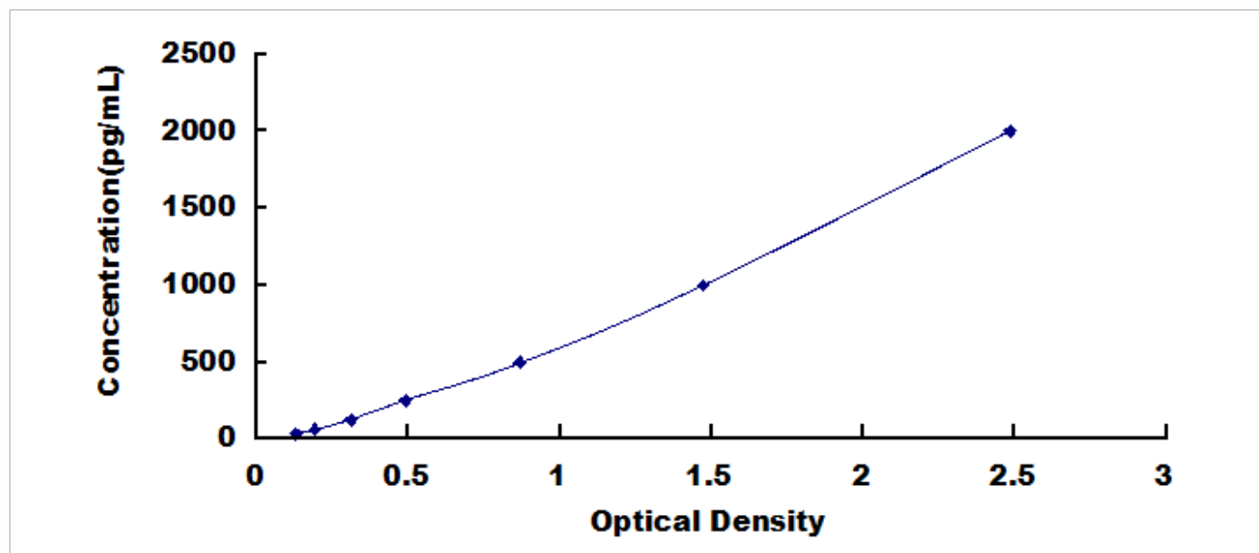
犬脑钠素(BNP)检测试剂盒标准曲线
