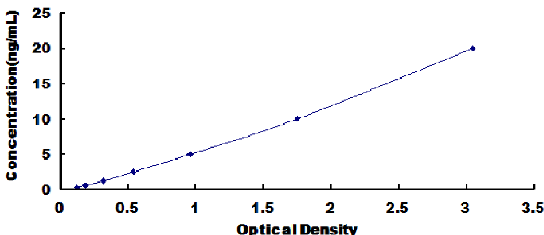
人 C-Mer 原癌基因酪氨酸激酶(MERTK)试剂盒标准曲线
