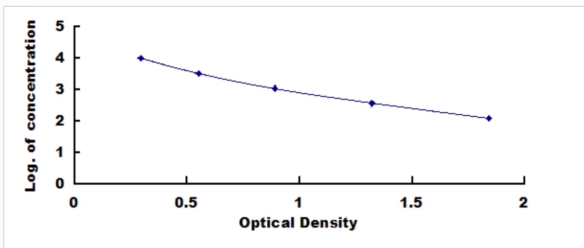
人 C-肽 (CP) 检测试剂盒标准曲线
