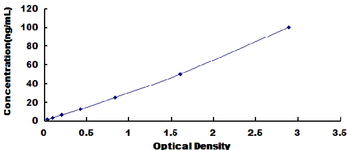
人 C4 结合蛋白 \alpha (C4BP \alpha ) 试剂盒标准曲线
