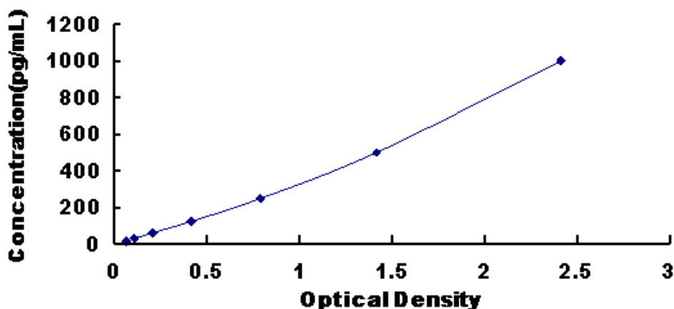
图 1: 人的降钙素(CT)试剂盒标准曲线
