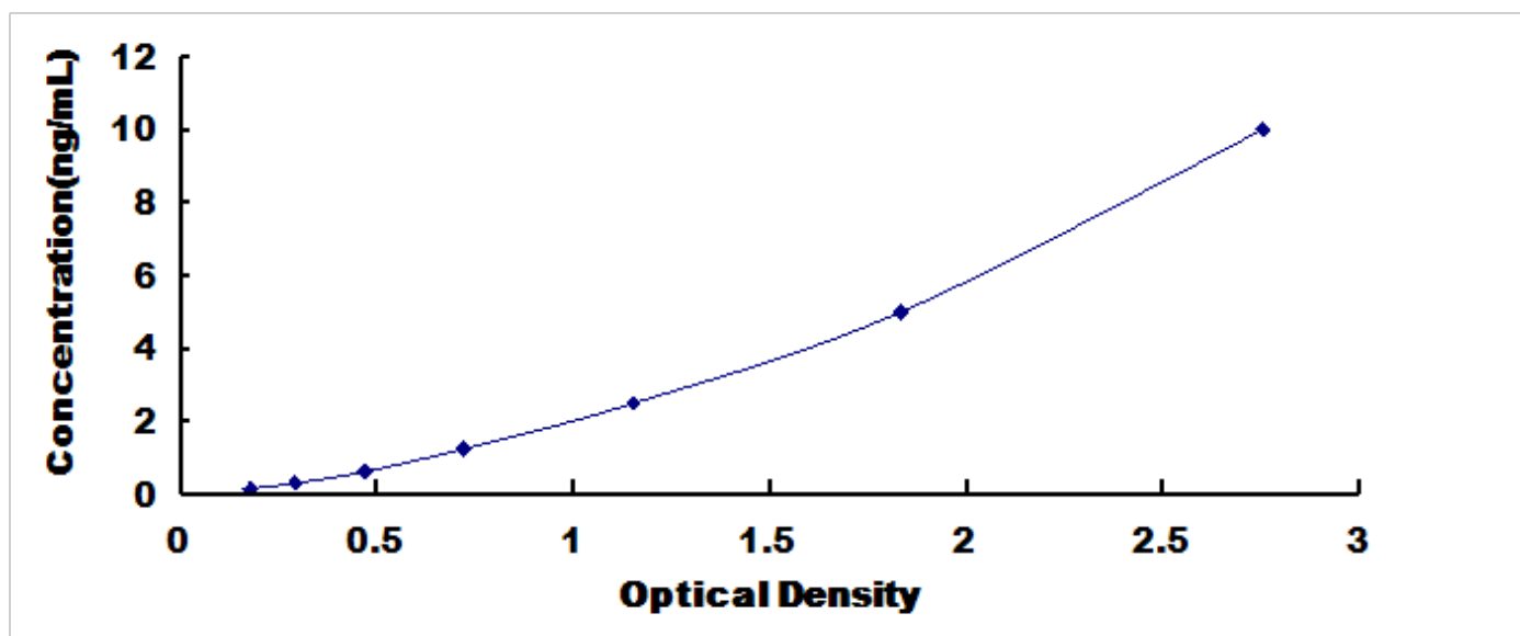
大鼠钙/钙调蛋白依赖性蛋白激酶 II \alpha (CAMK2 \alpha ) 检测试剂盒标准曲线
