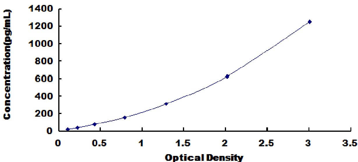
人癌胚抗原(CEA)检测试剂盒标准曲线
