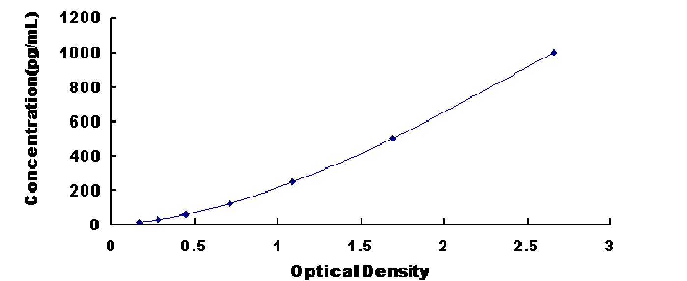
人心肌营养素 1(CT1)试剂盒标准曲线
