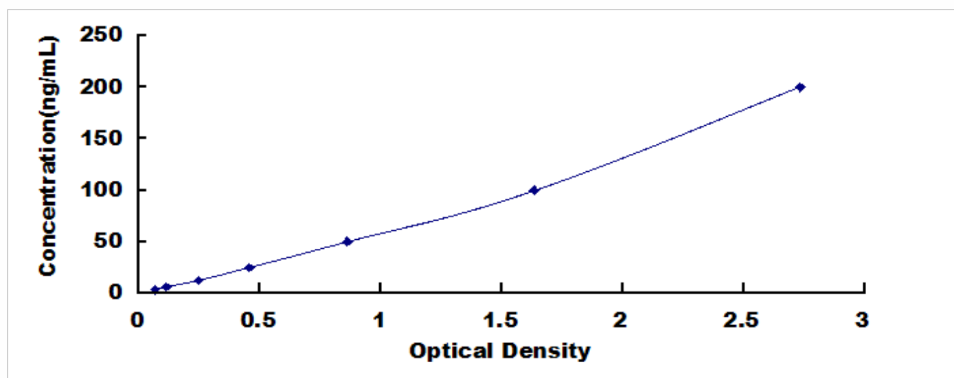
大鼠肉毒碱棕榈酰基转移酶 1A(CPT1A)检测试剂盒标准曲线
