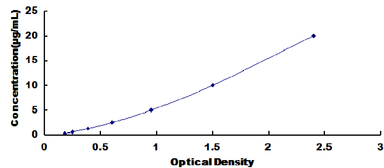
牛酪蛋白 \kappa (CSN3) 试剂盒标准曲线
