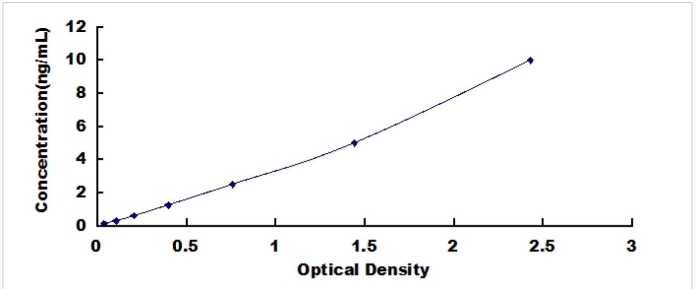
人胱天蛋白酶 14 (CASP14) 检测试剂盒标准曲线
