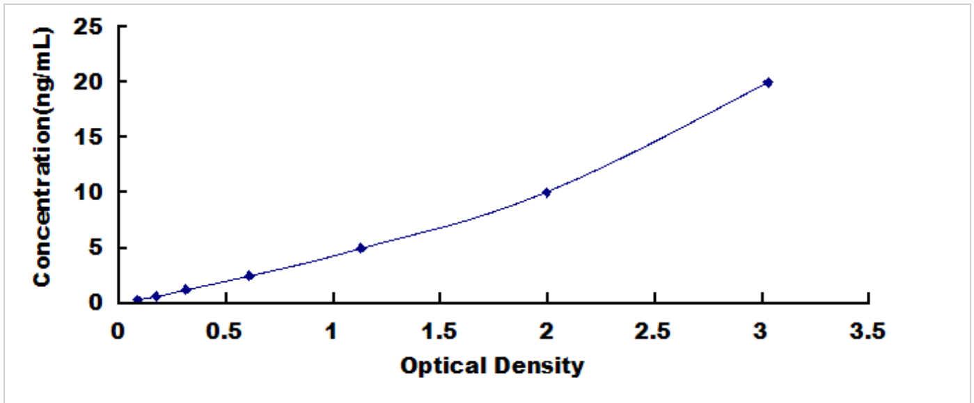
人胱天蛋白酶 9 (CASP9) 检测试剂盒标准曲线
