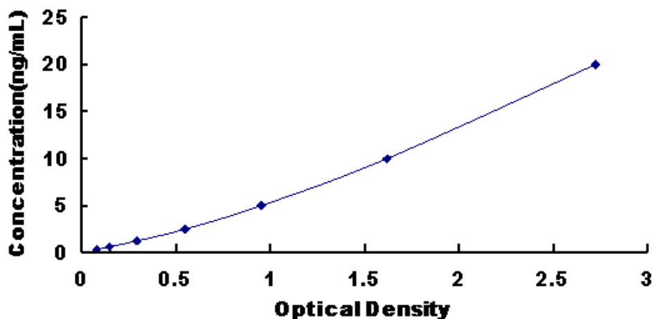
图 1: 大鼠过氧化氢酶(CAT)试剂盒标准曲线
