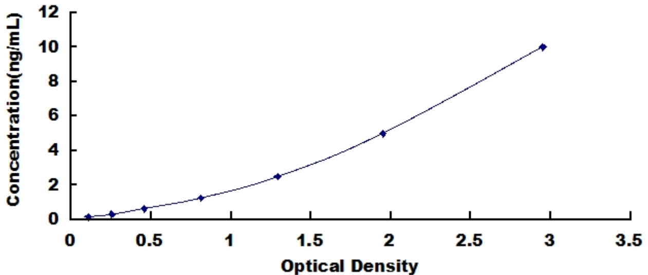
小鼠儿茶酚-O-甲基转移酶 (COMT) 检测试剂盒标准曲线
