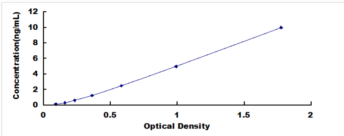
人组织蛋白酶 G (CTSG) 检测试剂盒标准曲线
