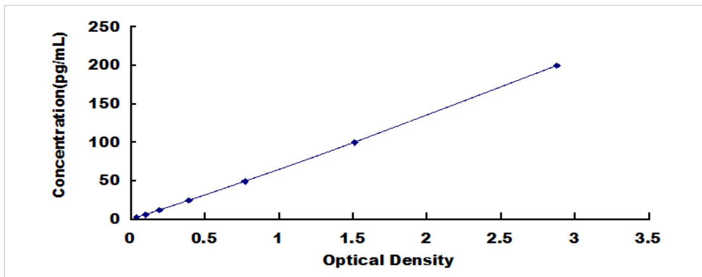
小鼠组织蛋白酶 G (CTSG) 检测试剂盒标准曲线
