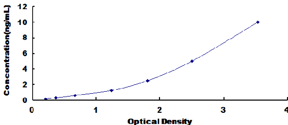
大鼠窖蛋白(CAV1)试剂盒标准曲线
