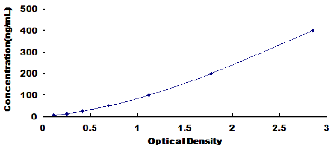
大鼠铜蓝蛋白(CP)试剂盒标准曲线
