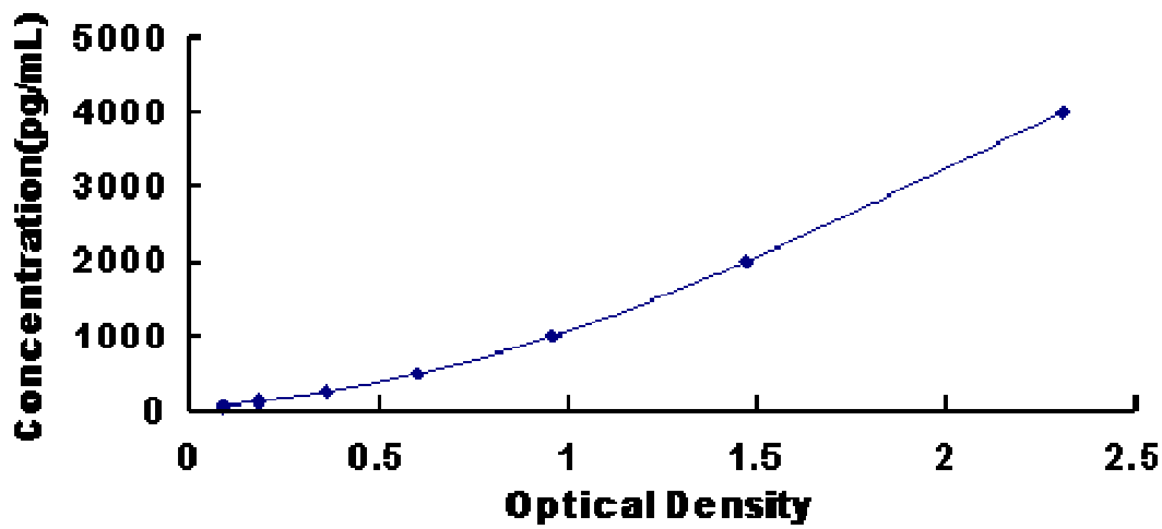
人夏科—雷登氏结晶蛋白(CLC)试剂盒标准曲线
