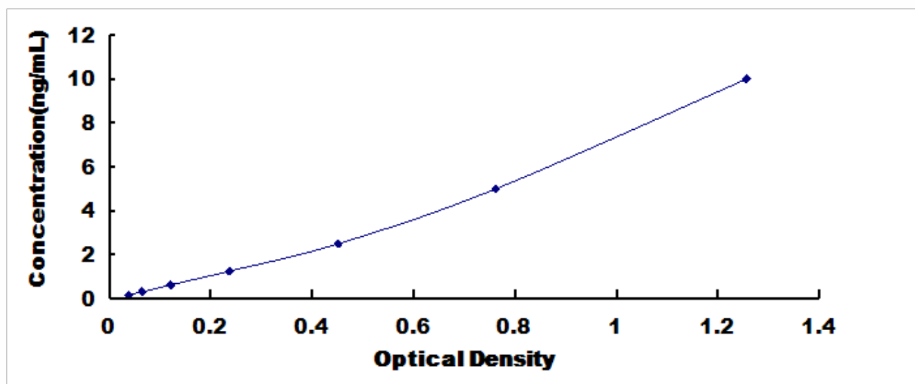
小鼠趋化因子 C-X3-C-基元配体 1 (CX3CL1) 检测试剂盒标准曲线
