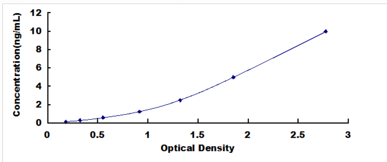
人趋化因子 C-X3-C-基元配体 1 (CX3CL1) 检测试剂盒标准曲线
