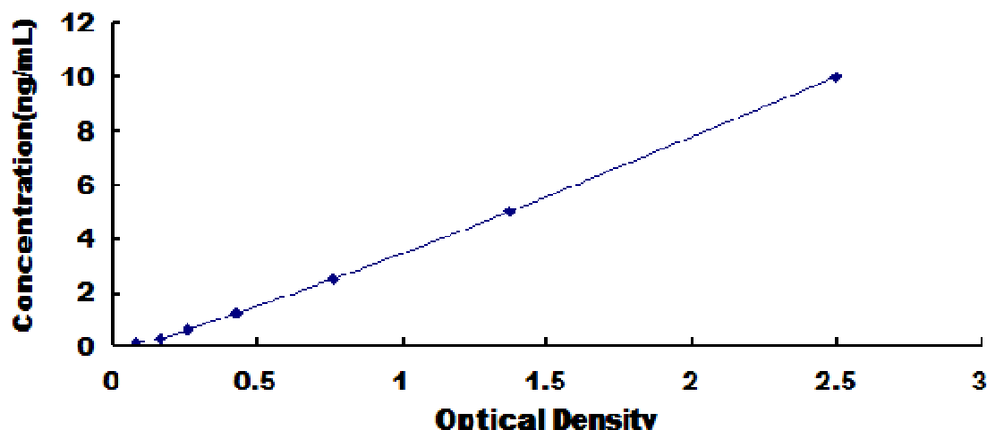
小鼠几丁质酶 1 (CHIT1) 检测试剂盒标准曲线
