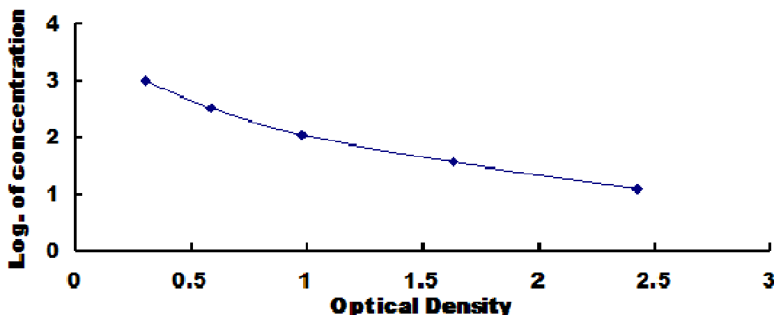
豚鼠胆囊收缩素八肽 (CCK8) 检测试剂盒标准曲线
