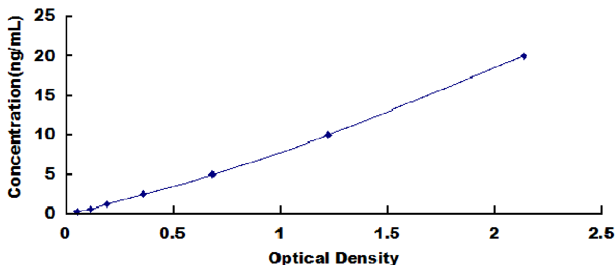
人烟碱型胆碱受体 \alpha 3 (CHRN \alpha 3) 试剂盒标准曲线
