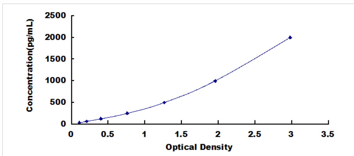
人封闭蛋白 5 (CLDN5) 检测试剂盒标准曲线
