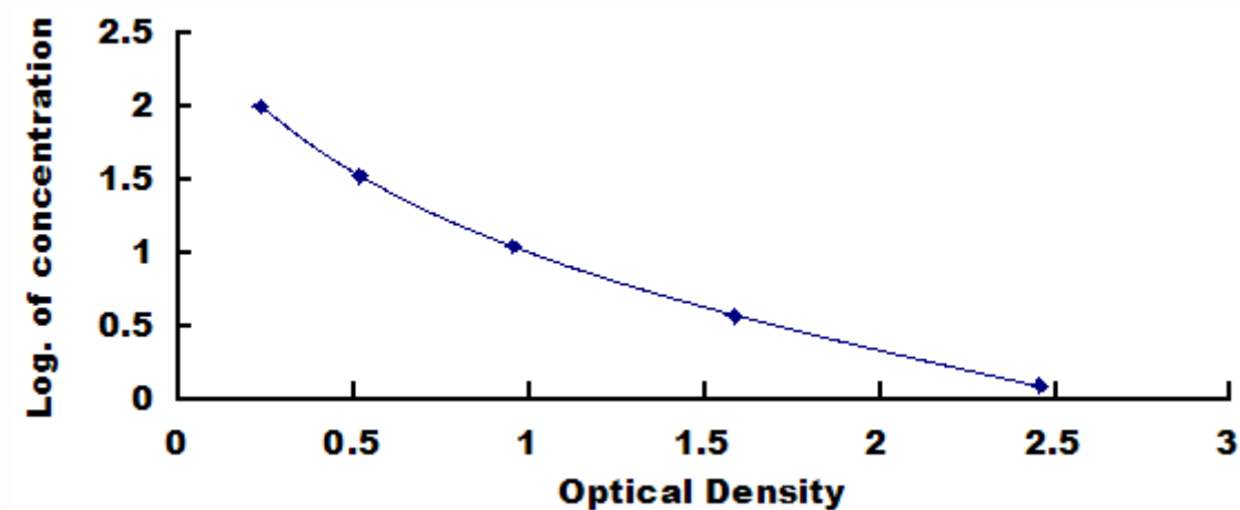
氯前列烯醇(CP)检测试剂盒标准曲线
