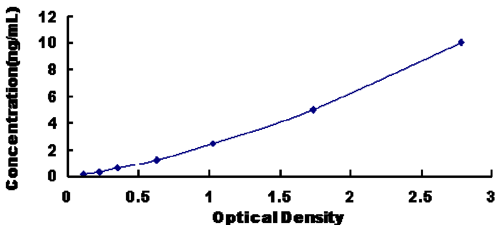
人 CD24 试剂盒标准曲线
