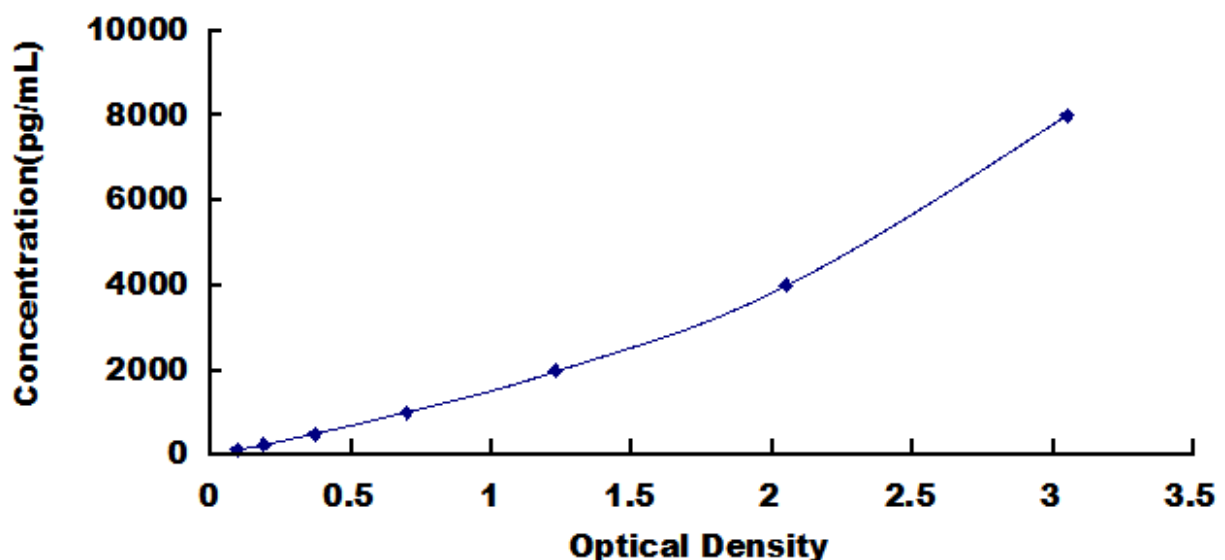
人凝血因子 V (F5) 检测试剂盒标准曲线
