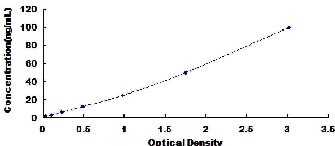
大鼠凝血因子 XⅢA1 肽(FXⅢA1)试剂盒标准曲线
