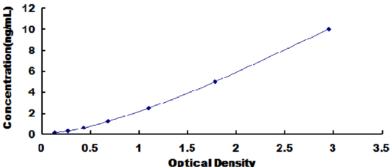
小鼠可卡因安非他明调节转录肽(CART)检测试剂盒标准曲线
