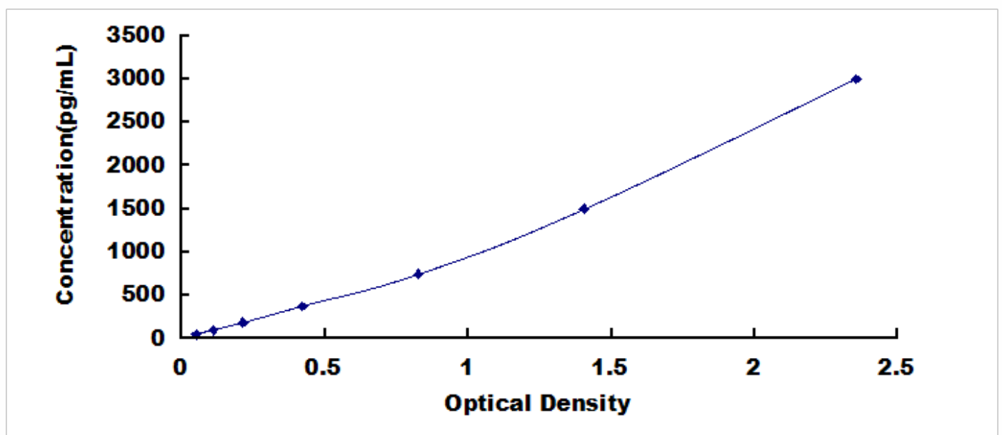
小鼠Ⅲ型胶原(COL3)检测试剂盒标准曲线
