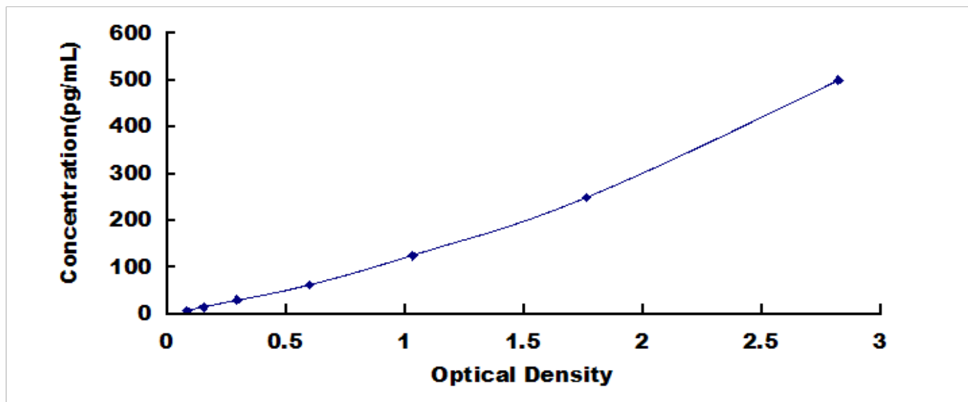
人巨噬细胞集落刺激因子(MCSF)检测试剂盒标准曲线
