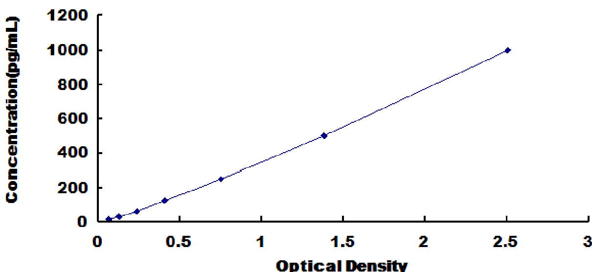
大鼠粒细胞巨噬细胞集落刺激因子 (GMCSF) 检测试剂盒标准曲线
