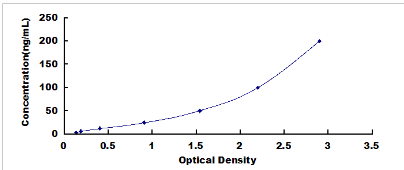
小鼠补体成分 3(C3)检测试剂盒标准曲线
