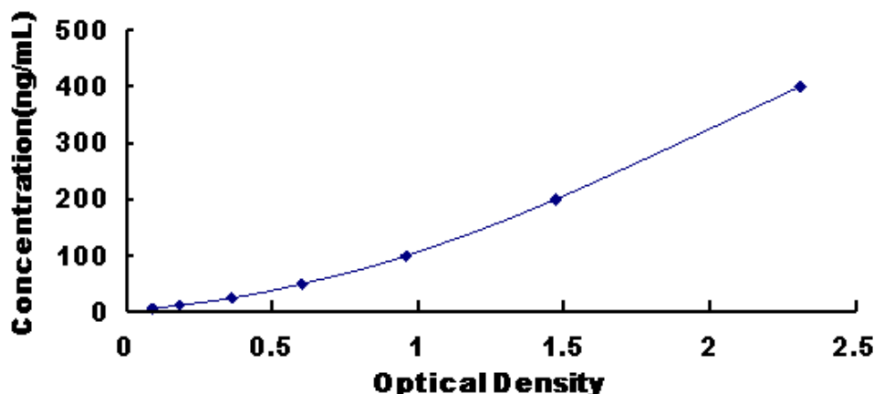
图 1: 犬的补体 3a(C3a)试剂盒标准曲线
