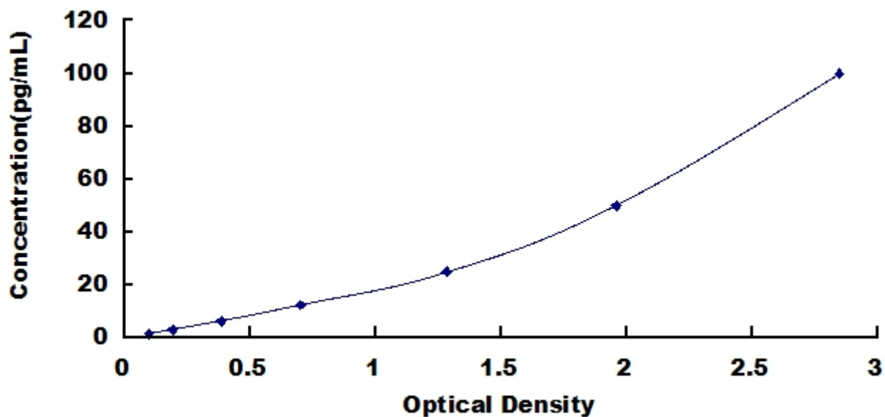
大鼠补体 3a (C3a) 检测试剂盒标准曲线
