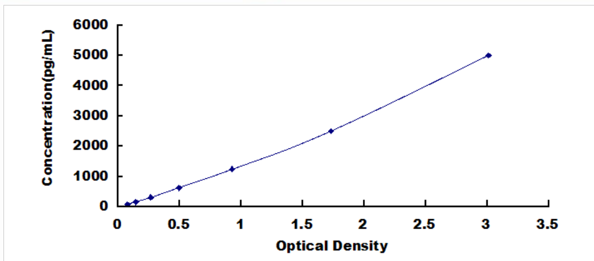
人补体 3a (C3a) 检测试剂盒标准曲线
