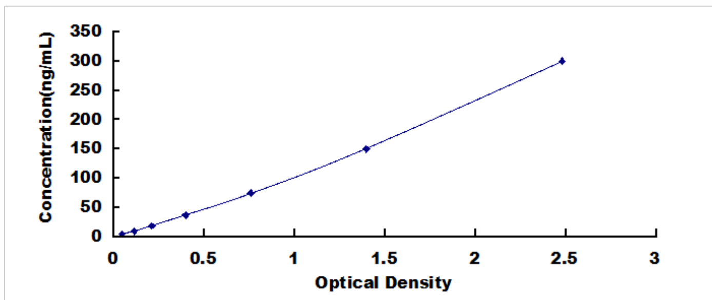
人补体成分 4d (C4d) 检测试剂盒标准曲线
