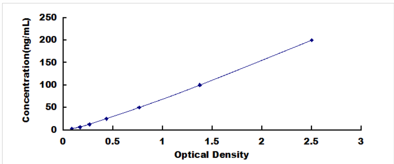
犬补体成分 5a (C5a) 检测试剂盒标准曲线
