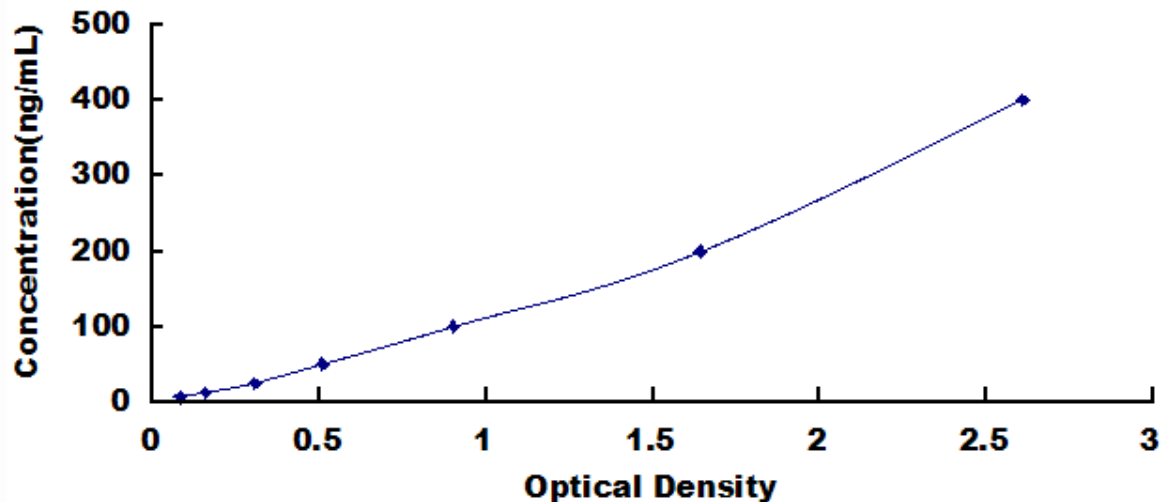
人补体成分 7 (C7) 试剂盒标准曲线
