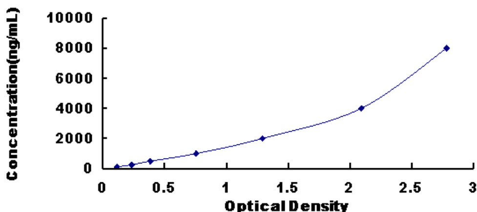
图 1: 大鼠补体因子 H(CF-H)试剂盒标准曲线
