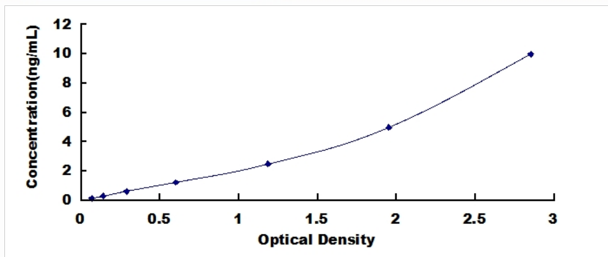
人补体因子 I (CFI) 检测试剂盒标准曲线
