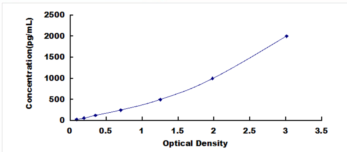
小鼠结缔组织生长因子 (CTGF) 检测试剂盒标准曲线
